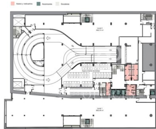
Sótano -1
